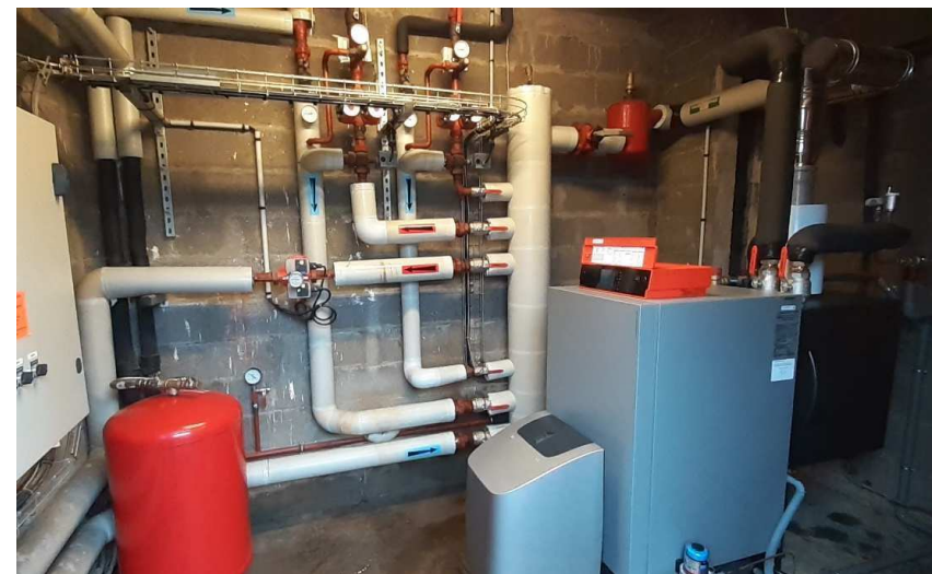
Nouvelle chaufferie
